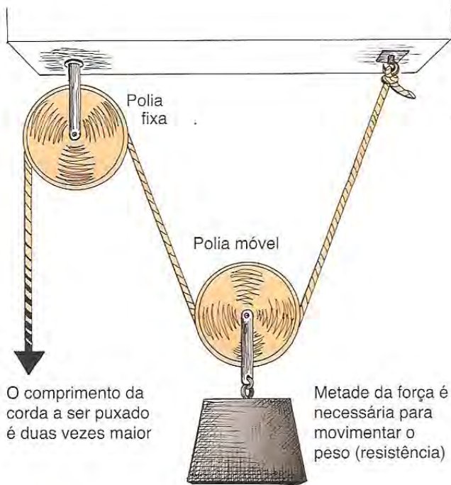
Figura 8.34 A polia móvel tem uma vantagem mecânica para força.
