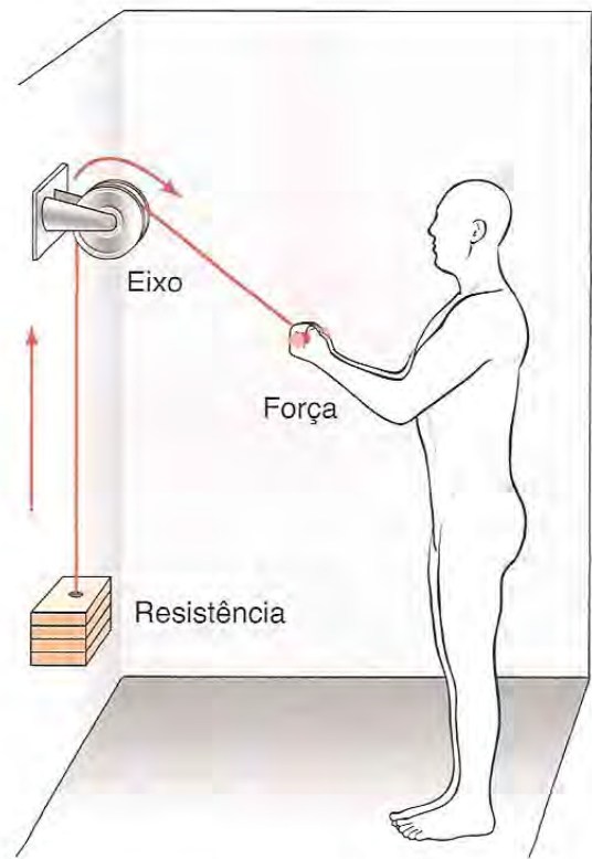
Figura 8.32 Polia fixa. O seu objetivo é mudar a direção da força.
