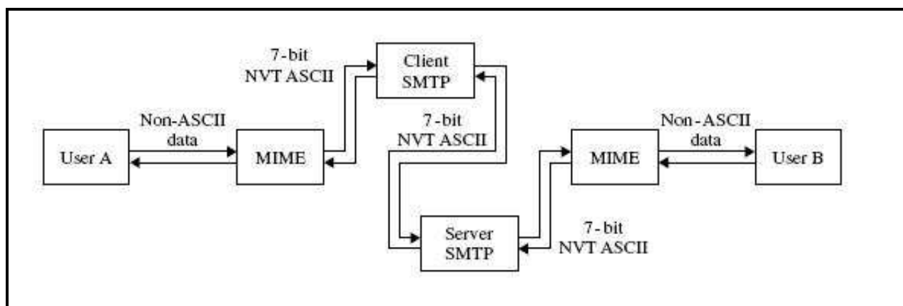
Figura 10 – Uso do MIME em conjunto com o protocolo SMTP
