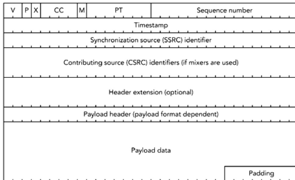
Figura 12 – Cabeçalho do protocolo RTP.
