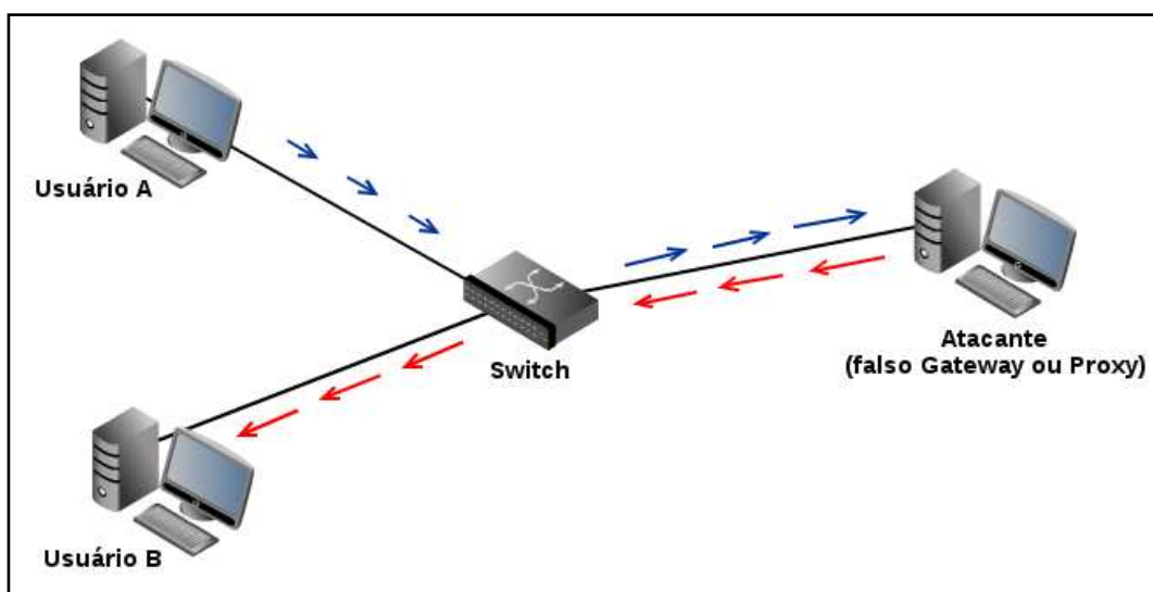
Figura 8 – O famoso ataque Man in the Middle
