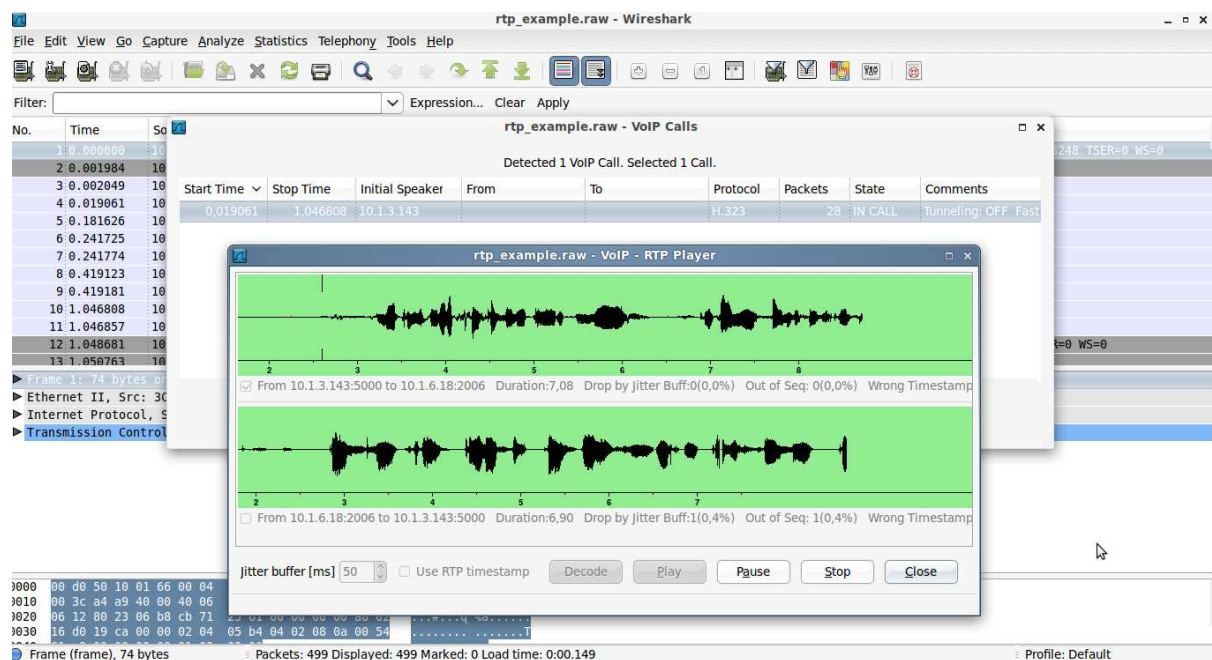
Figura 5 – Captura, detecção, decodificação e reprodução de chamada VoIP
