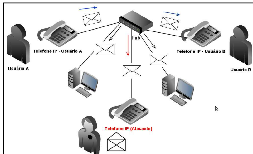
Figura 7 – Call Eavesdropping em redes utilizando hubs
